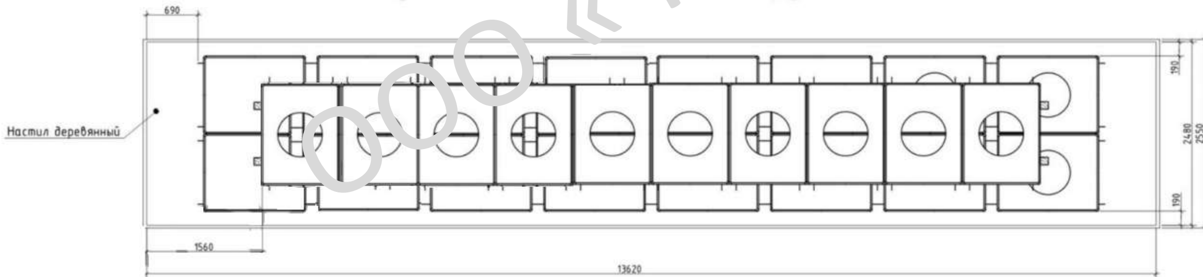
Кузов шторного полуприцепа (вид сверху)
