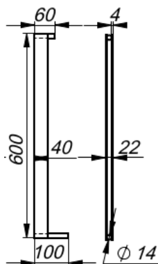
Рис. 8. Габариты кронштейнов ККПр-60 (вид сбоку и спереди).
