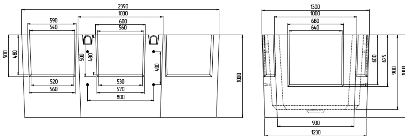
Рис. 7. Габариты нижнего элемента колодца (вид сбоку и с торца элемента).
