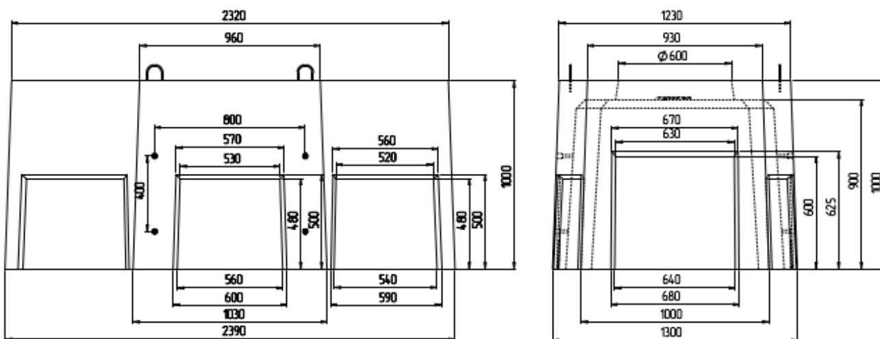
Рис. 6. Габариты верхнего элемента колодца (вид сбоку и с торца элемента).
