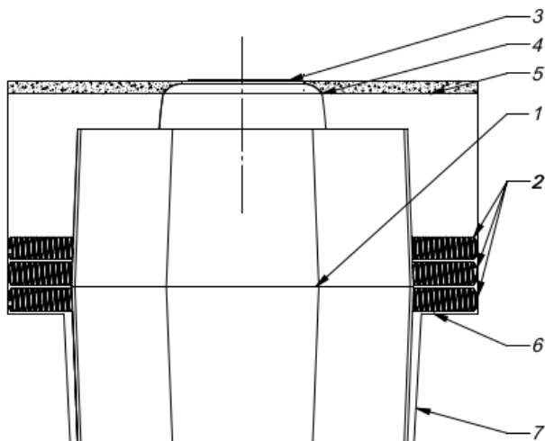
Рис. 2. Схема смонтированного «ККСр-4-10 ГЕК-У гидро» как подземного сооружения: 1 – элементы колодца в сборе; 2 – вводимые каналы трубопровода «СПИРАПАЙП™»; 3 – люк ГТС; 4 – бетонная обмазка горловины; 5 – уровень грунта или дорожного покрытия; 6 – дно траншеи; 7 – пазуха котлована.
