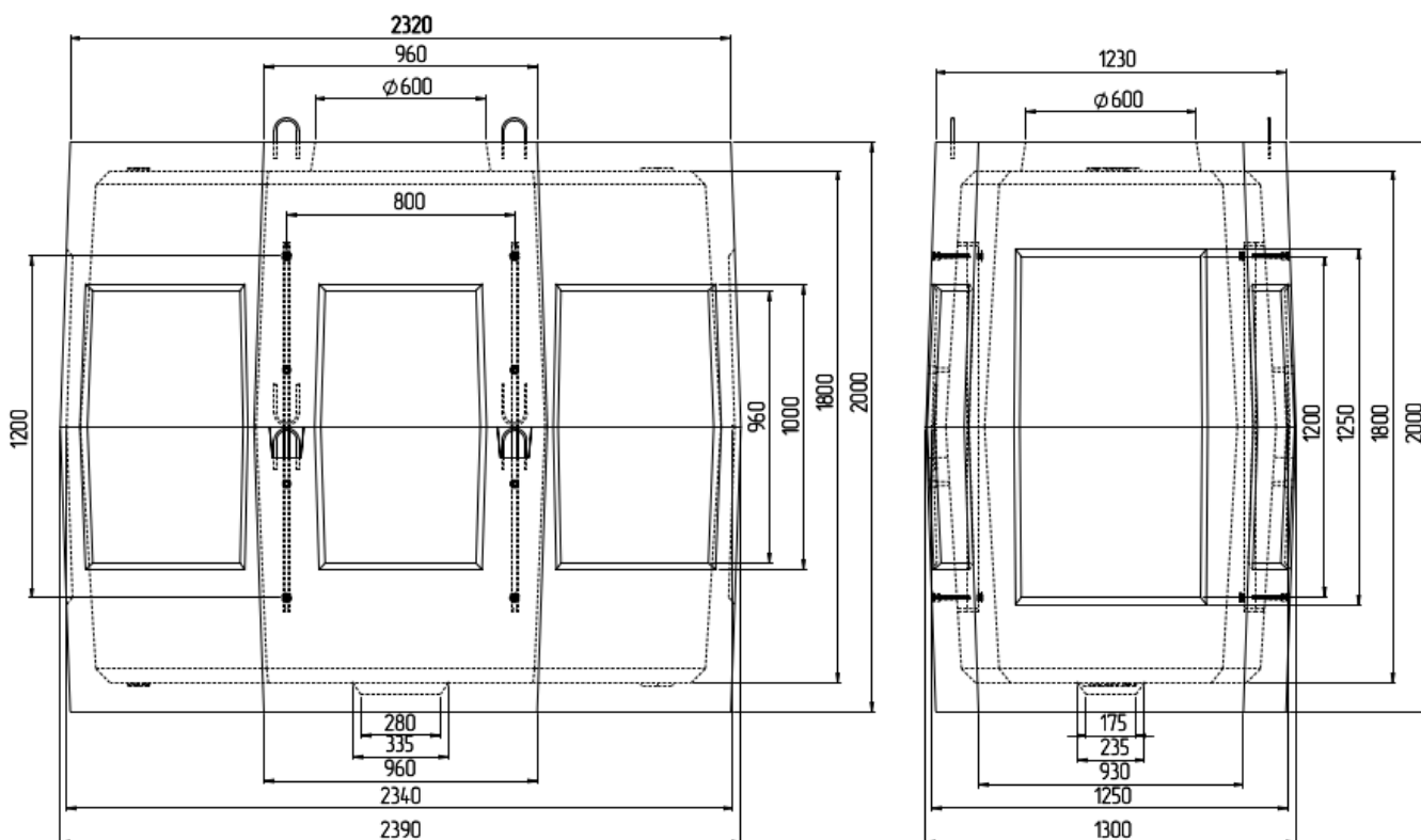
Рис. 9. Габариты колодца «ККСр-4-10 ГЕК-У гидро» в сборе (вид сбоку и спереди).
