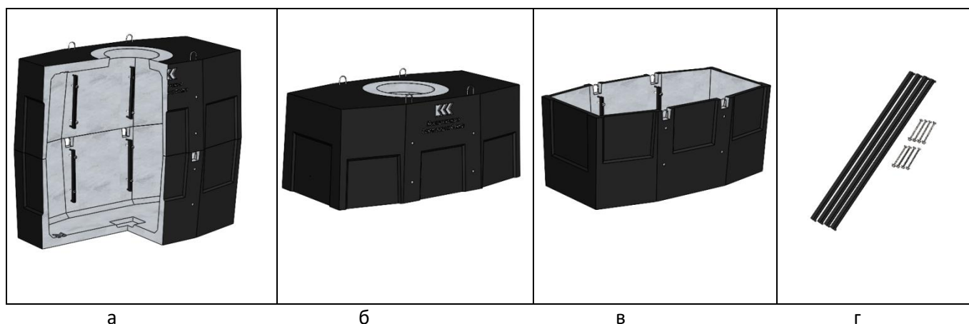
Рис. 1. Колодец «ККСр-4-10 ГЕК-У КСС (В25)» в одно и двухслойной гидроизоляции: а – как изделие в сборе до монтажа; б – верхний элемент; в – нижний элемент; г – комплект устанавливаемого оснащения.
