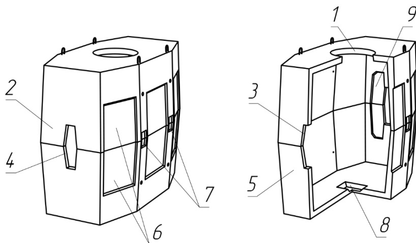
Рис. 4. Колодец «ККСр-4-80», внешний вид и детали элементов колодца: 1 – круглое отверстие для люка; 2 – верхний элемент; 3 – технологическое отверстие верхнего элемента; 4 – технологическое отверстие нижнего элемента; 5 – нижний элемент; 6 – ниши на наружных поверхностях боковых стен; 7 – гнезда с подъёмными петлями на нижнем элементе; 8 – приямок для стока воды; 9 – участок с тонкими неармированными стенками вокруг технологических отверстий.
