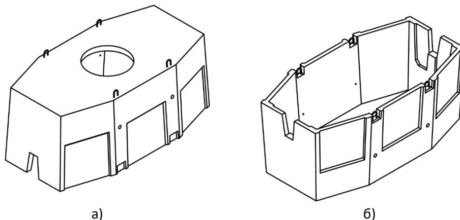
Рис. 1. Колодец «ККСр-4-80» как изделие: а – верхний элемент; б – нижний элемент.
