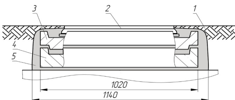
Рис. 14 Диаметры колец и обмазанной бетоном горловины при использовании пары «КО-ЧП» и «КО-Ч»: 1 – уровень земли на газоне, асфальта на тротуаре; 2 – люк лёгкого типа; 3 – кольцо «КО-Ч»; 4 – кольцо «КО-ЧП»; 5 - обмазка горловины бетоном со щебнем.
