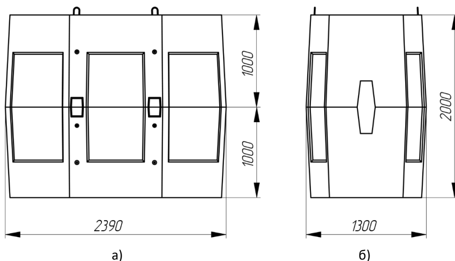
Рис. 5. Габаритные размеры колодца «ККСр-4-80»: а - вид сбоку; б – вид с торца.
