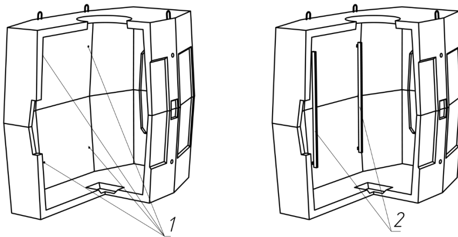
Рис. 3.1. Установка кронштейнов «ККП-130» на боковой стене колодца «ККСр-4-80»: 1 – отверстия для ершей в стене колодца; 2 – кронштейны «ККП-130» .
