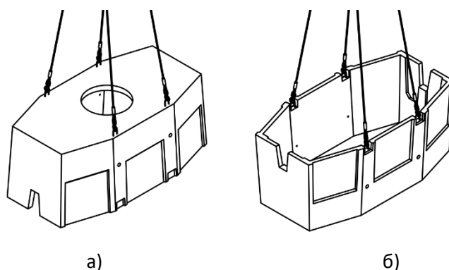
Рис. 9. Строповка элементов «ККСр-4-80»: а – верхнего элемента; б – нижнего элемента.
