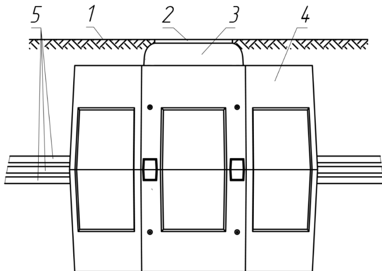
Рис. 2. Колодец «ККСр-4-80» как подземное асфальта; 2 – чугунный люк тяжелого типа; 3 – горловина в бетонной обмазке; 4 – корпус колодца в сборе; 5 – вводимые каналы, 12 труб.
