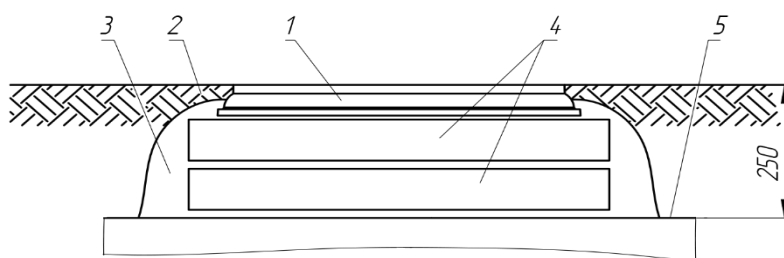
Рис. 12. Расстояние от перекрытия колодца до уровня земли (асфальта) на тротуаре и газоне должно быть – не менее 250 мм: 1 – люк чугунный; 2 – уровень земли на газоне, асфальта на тротуаре; 3 – обмазка горловины бетоном со щебнем; 4 – опорные кольца типа КО; 5 – перекрытие колодца «ККСр-4-10».
