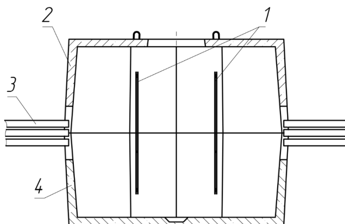
Рис. 10. Ввод труб в колодец «ККСр-4-80»: 1 – кронштейны ККП-130; 2 - торцевая стена верхнего элемента колодца; 3 – ввод хризотилцементных труб в проёмы в торцевых стенах элементов колодца; 4 – торцевая стена нижнего элемента колодца.
