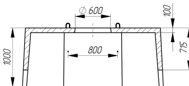
Рис. 8. Размеры колодца «ККСр-4-80» на продольном разрезе верхнего элемента: толщина перекрытия; расстояние от перекрытия до технологического отверстия; диаметр горловины; расстояние между отверстиями для ершей.
