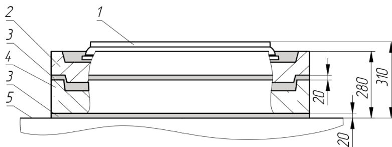
Рис. 13. Высота горловины с парой колец КО-ЧП и КО-Ч: 1 – люк чугунный лёгкого типа; 2 – кольцо «КО-Ч»; 3 – слои бетона; 4 – опорное кольцо «КО-ЧП»; 5 – перекрытие колодца «ККСр-4-80»
