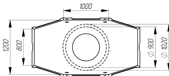
Рис. 6. Размеры перекрытия колодца «ККСр-4-80» с указанием диаметров опорных колец: 900 мм – кольца типа КО; 1020 мм – кольца КО-ЧП и КО-Ч.
